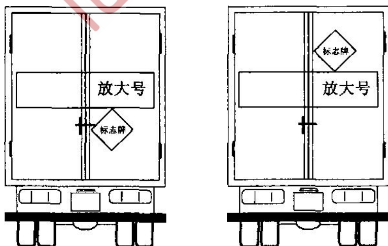
图 C.2 厢式车辆标志牌悬挂位置
