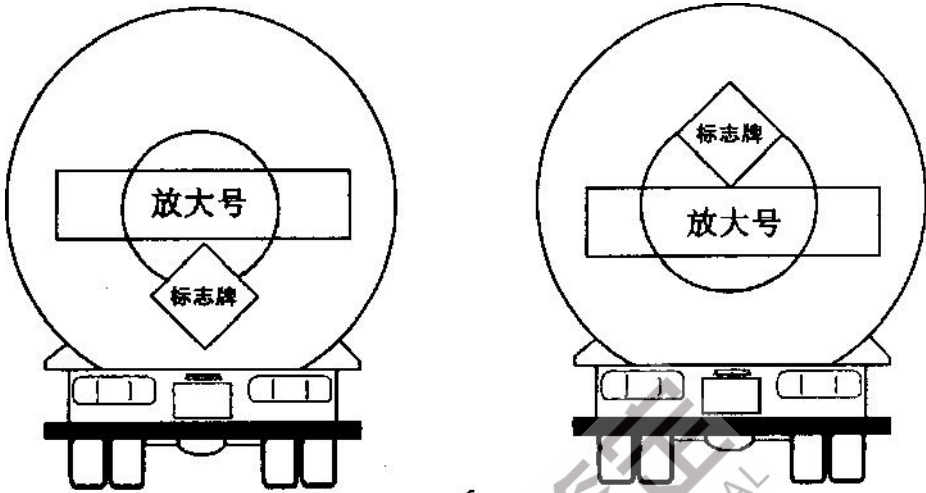
图 C.3 罐式车辆标志牌悬挂位置
